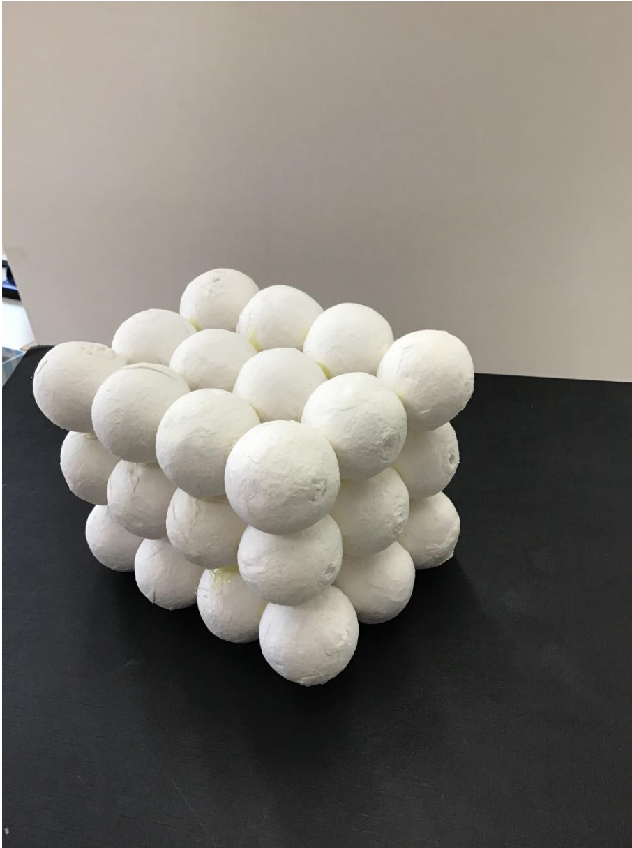
Teilchenmodell
